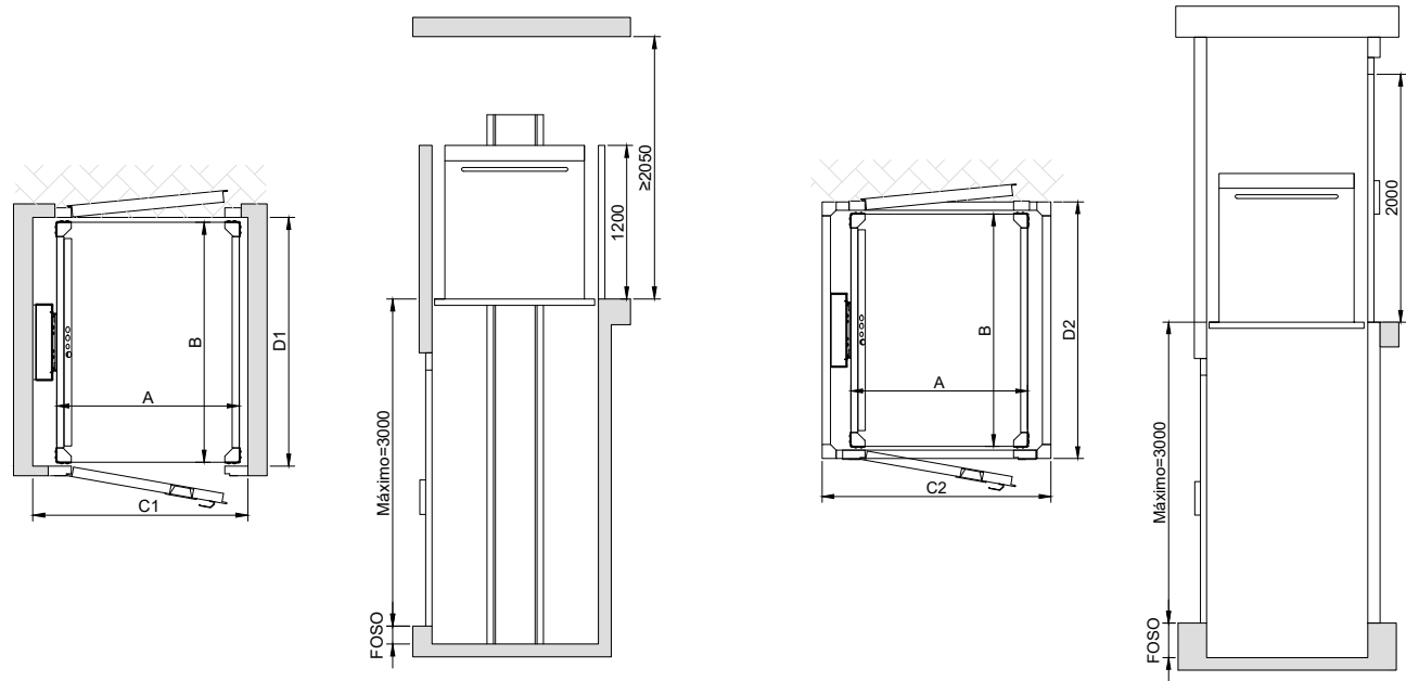
Cerramiento hueco en acero inox. y cristal por cuenta del cliente.
